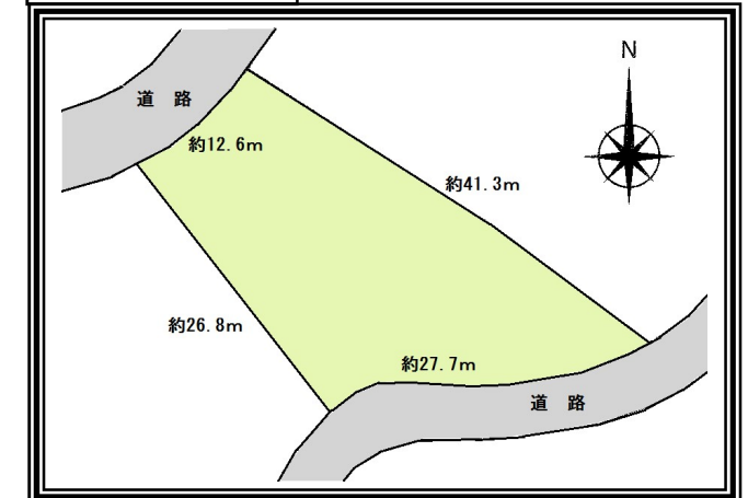
【敷地図】
