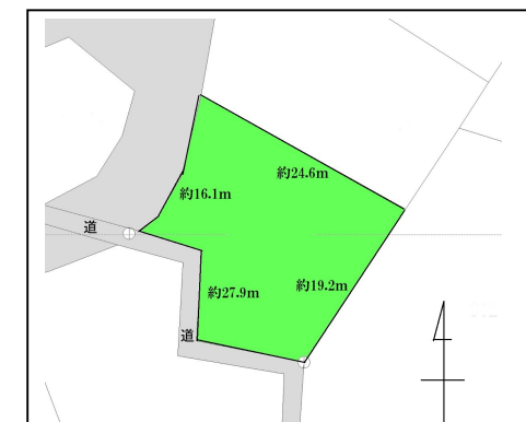
【公図】
