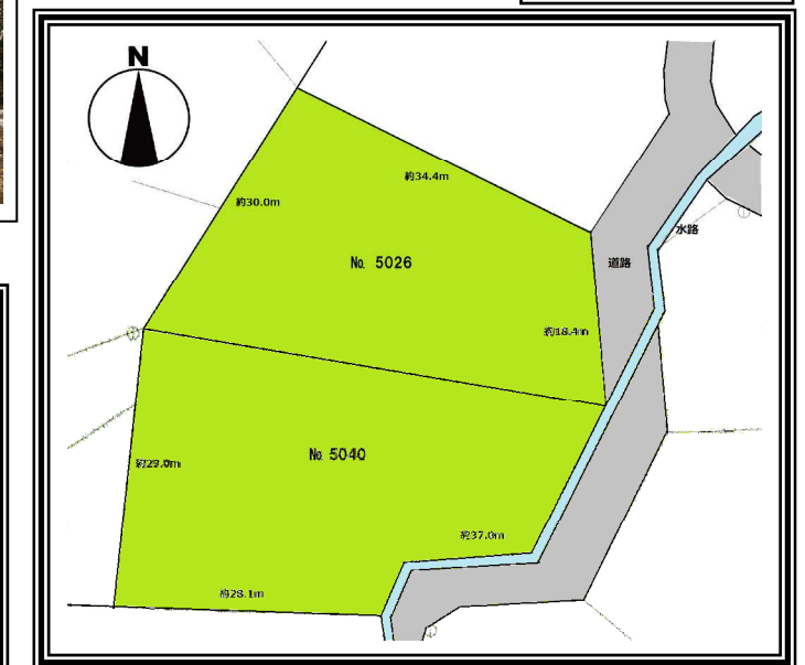
【敷地図】
