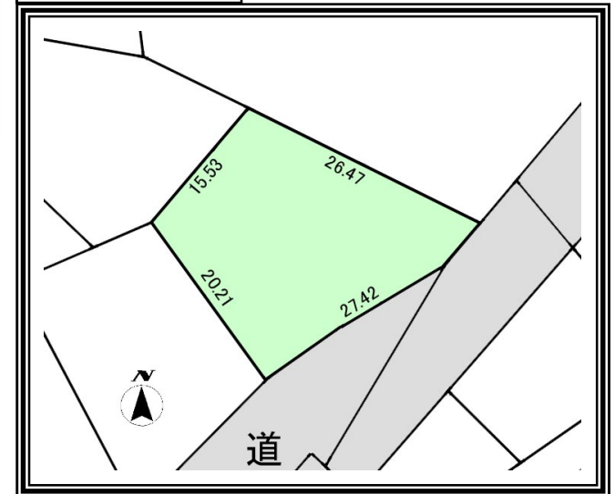
【敷地図】
