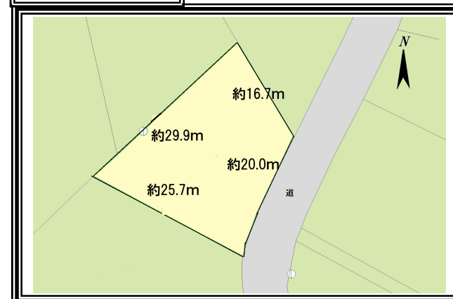
【敷地図】
