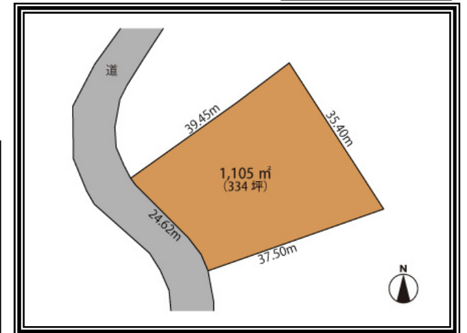
【敷地図】
