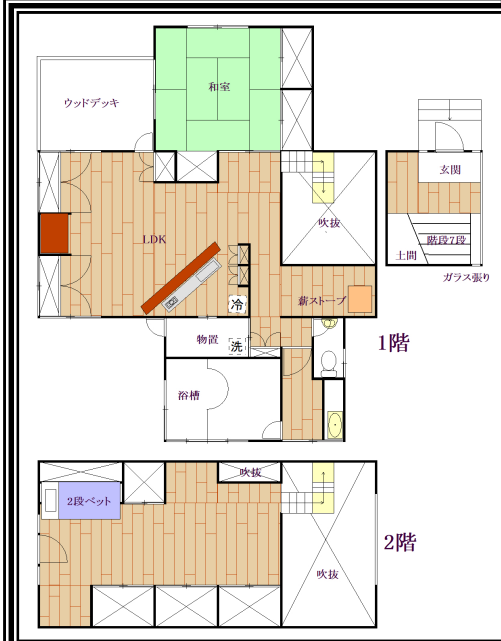
【間取り図】
