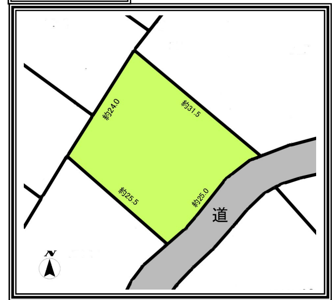
【敷地図】
